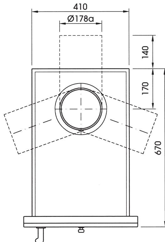
Draufsicht M 1:10
