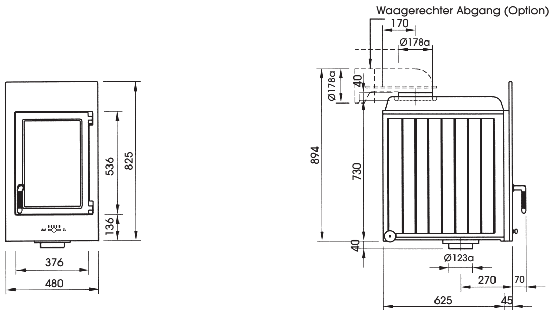
Ansicht
