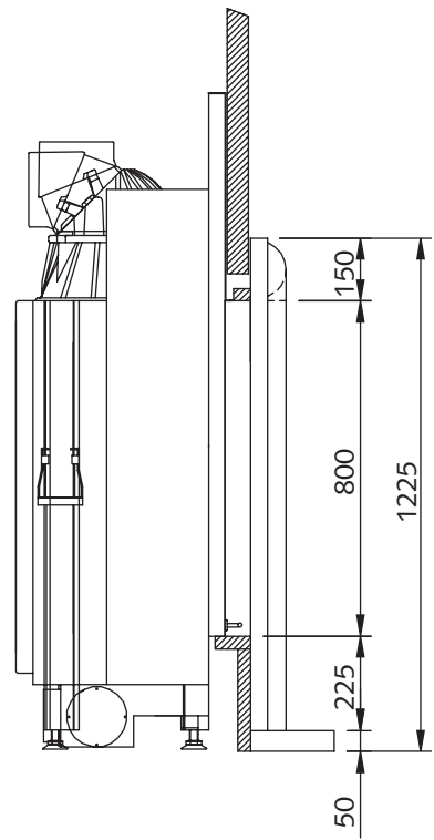
Seitenansicht
