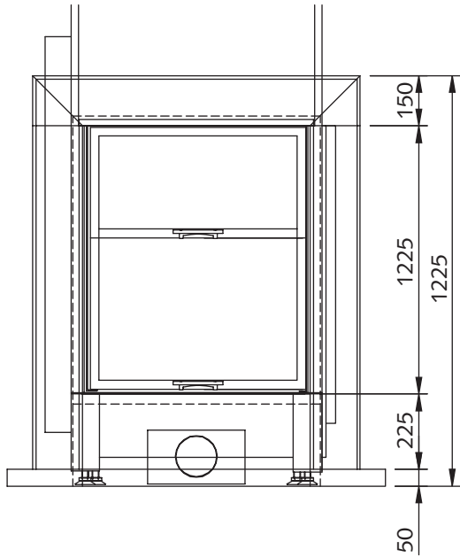
Ansicht
