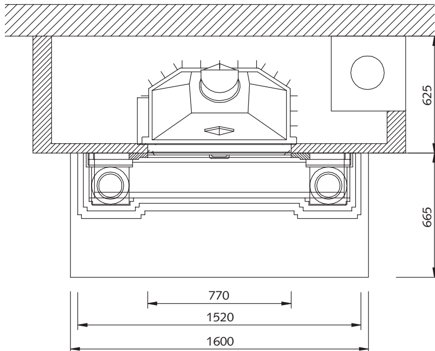
Draufsicht
