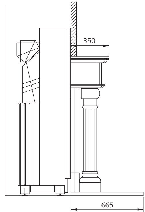
Seitenansicht
